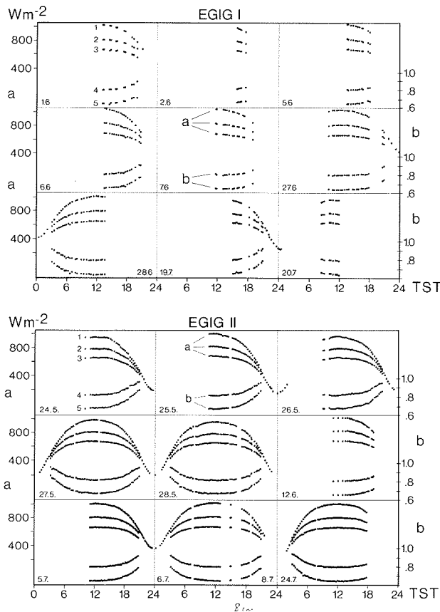
Abb. 3: Tagesgänge der Strahlungsströme (a) und der Quotienten der einzelnen Strahlungsströme (b). 1 = Gesamtstrahlung (J), 2 = J(OG1) , 3 = J(RG2) , 4 = J(OG1)/J , 5 = J(RG2)/J . Für (a) gilt die linke Skala, für (b) die rechte Skala.
