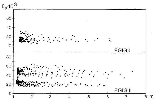
Abb. 5: Abhängigkeit des druckkorrigierten Ångströmschen Trübungskoeffizienten \beta_p von der optischen Luftmasse. Auswertung nach dem IGY-Instruction Manual (1958).
