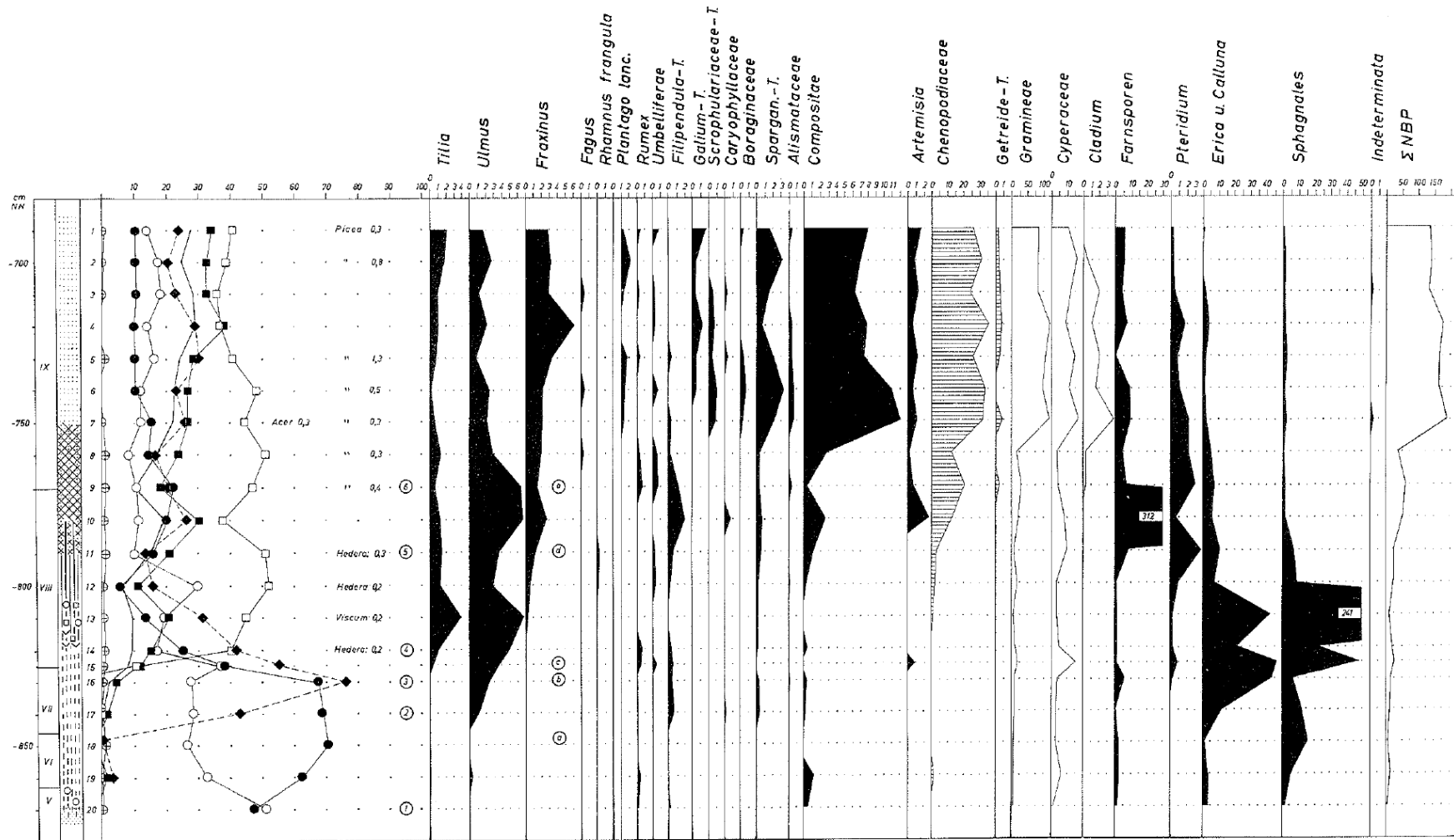
Abb. 8: Profil Ockholm-II (O-II) – Basistorf.
