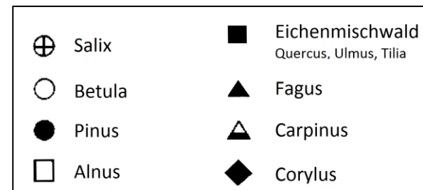
Abb. 10a: Profil Ockholm-I (O-I) – Baumpollen. „Schwarze Schnur“ und Teil des „Upper Peat“. Über dem Torf der „Schwarzen Schnur“ liegen etwa 120 cm Klei
