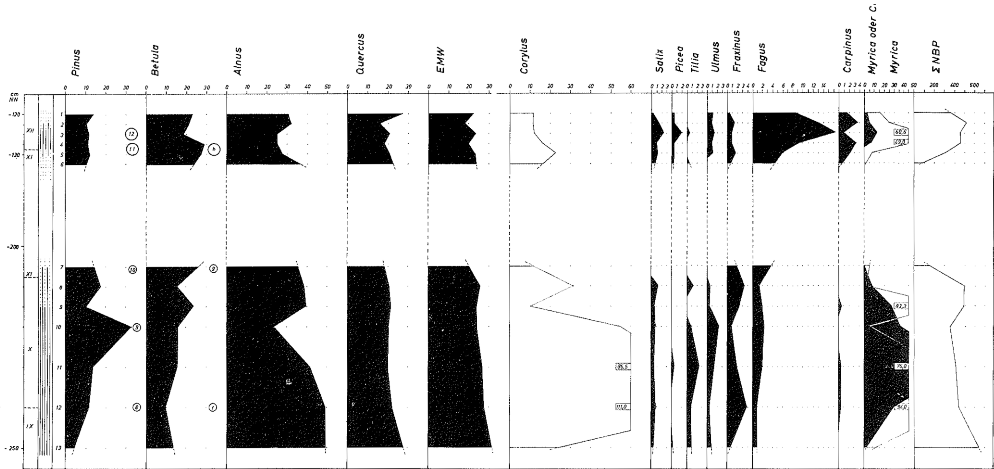
Abb. 10a: Profil Ockholm-I (O-I) – Baumpollen. „Schwarze Schnur“ und Teil des „Upper Peat“. Über dem Torf der „Schwarzen Schnur“ liegen etwa 120 cm Klei
