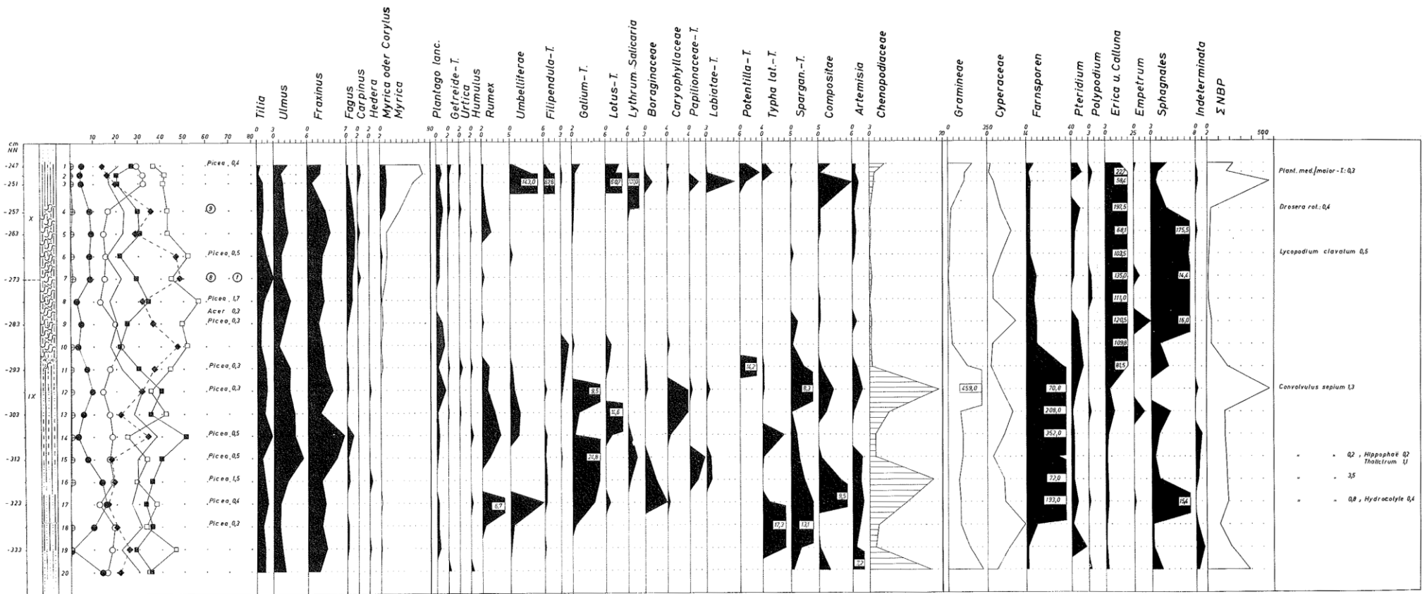
Abb. 12: Profil Bongsiel-II (B-II) – „Upper Peat“
