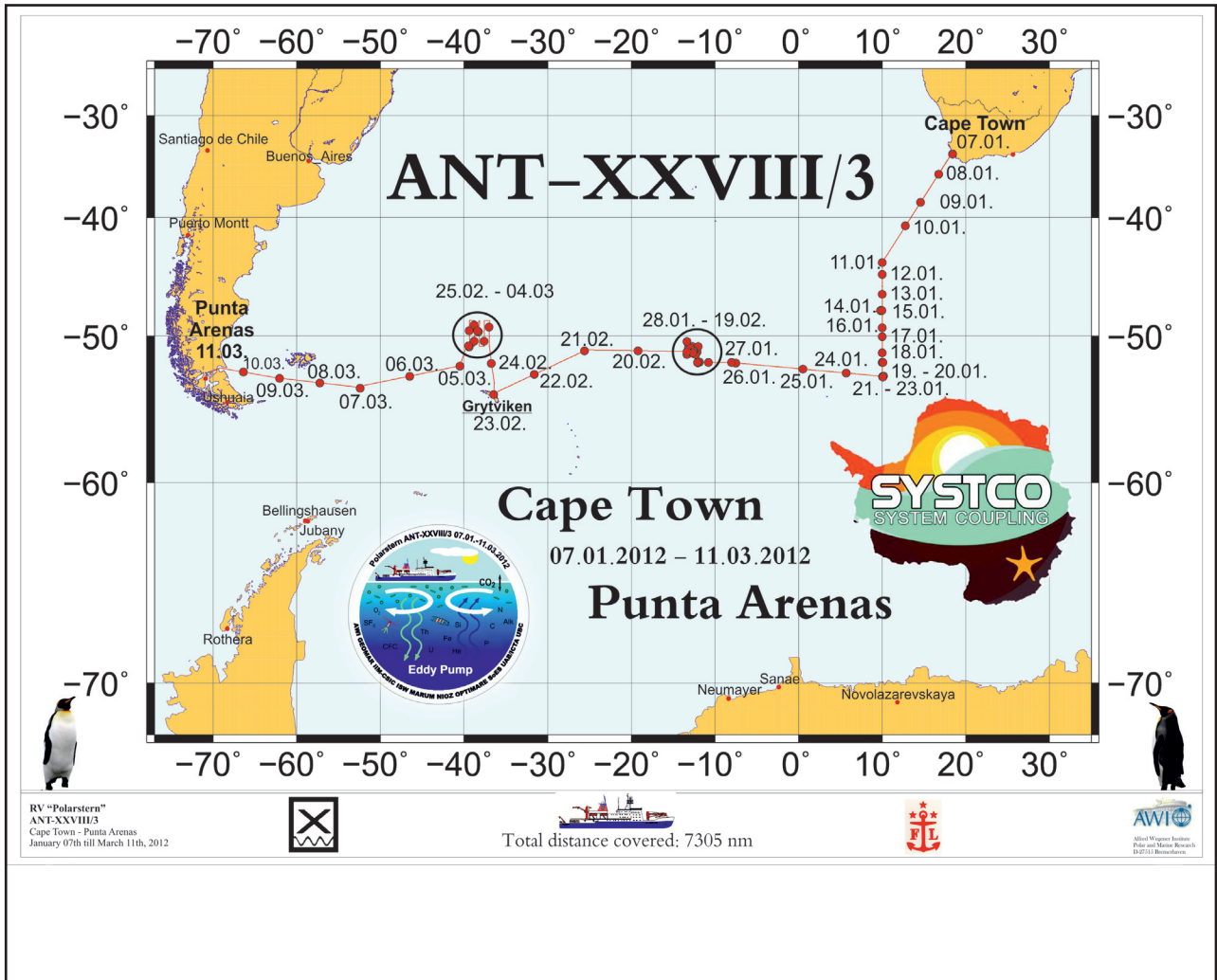
Abb. 1: Fahrtverlauf Polarstern-Expedition ANT-XXVIII/3
