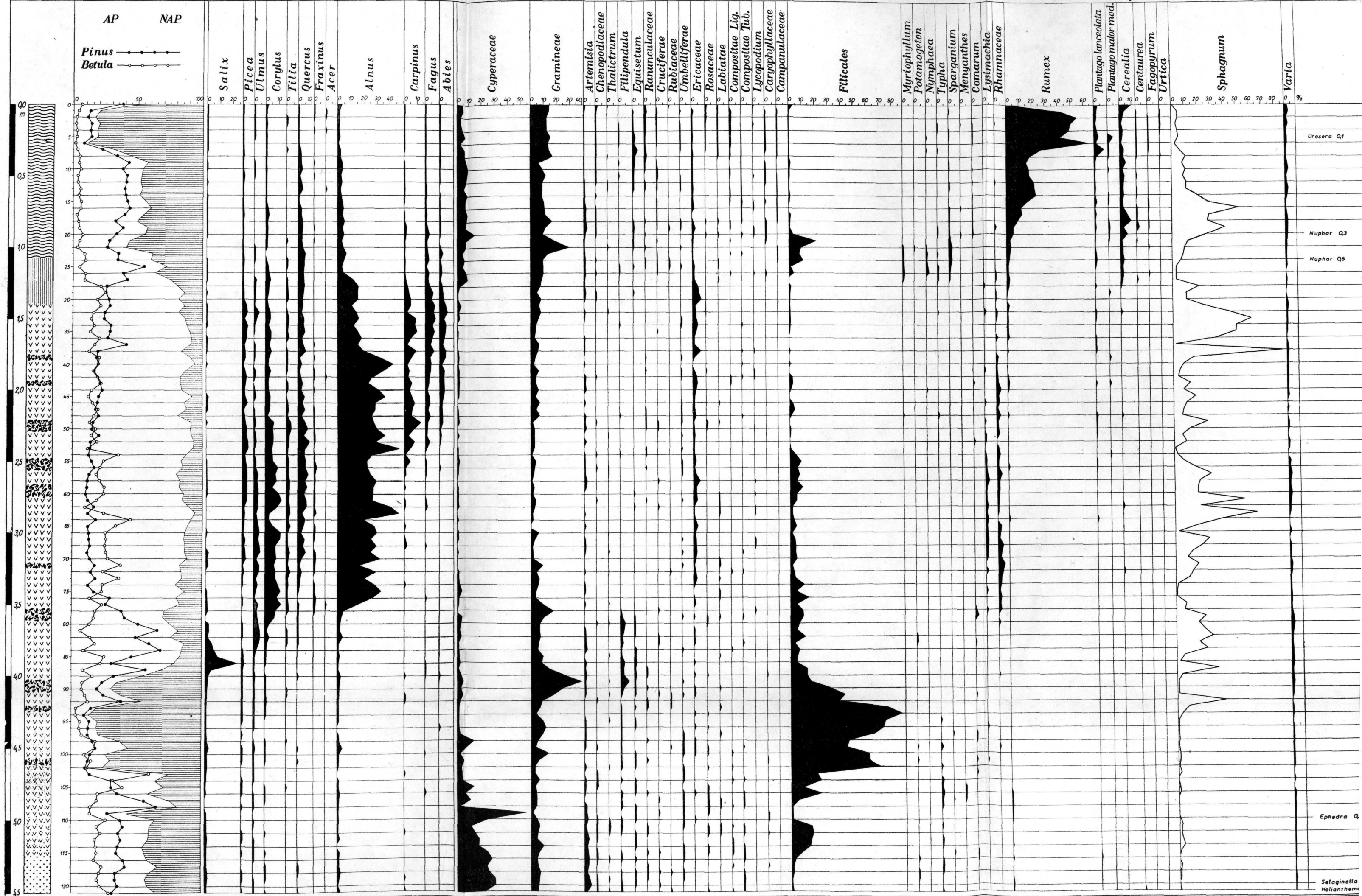
Ryc. 7. Diagram pyłkowy torfowiska Słopiec (250 m n.p.m.)
