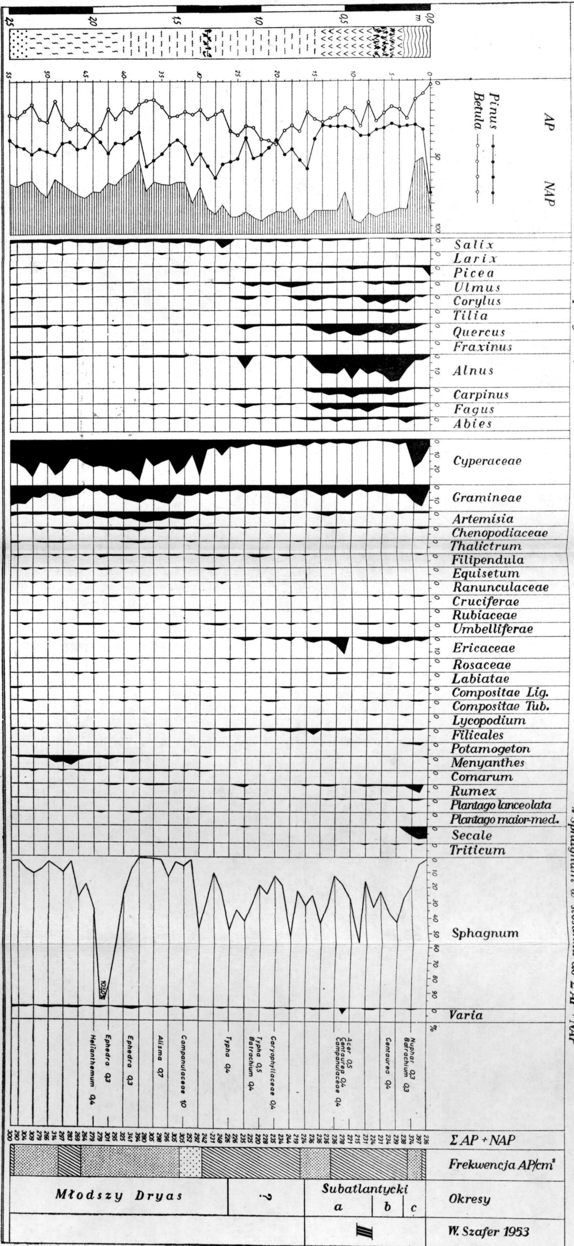
Ryc. 6. Diagram pyłkowy torfowiska Kawęczyn (180 m n.p.m.)
