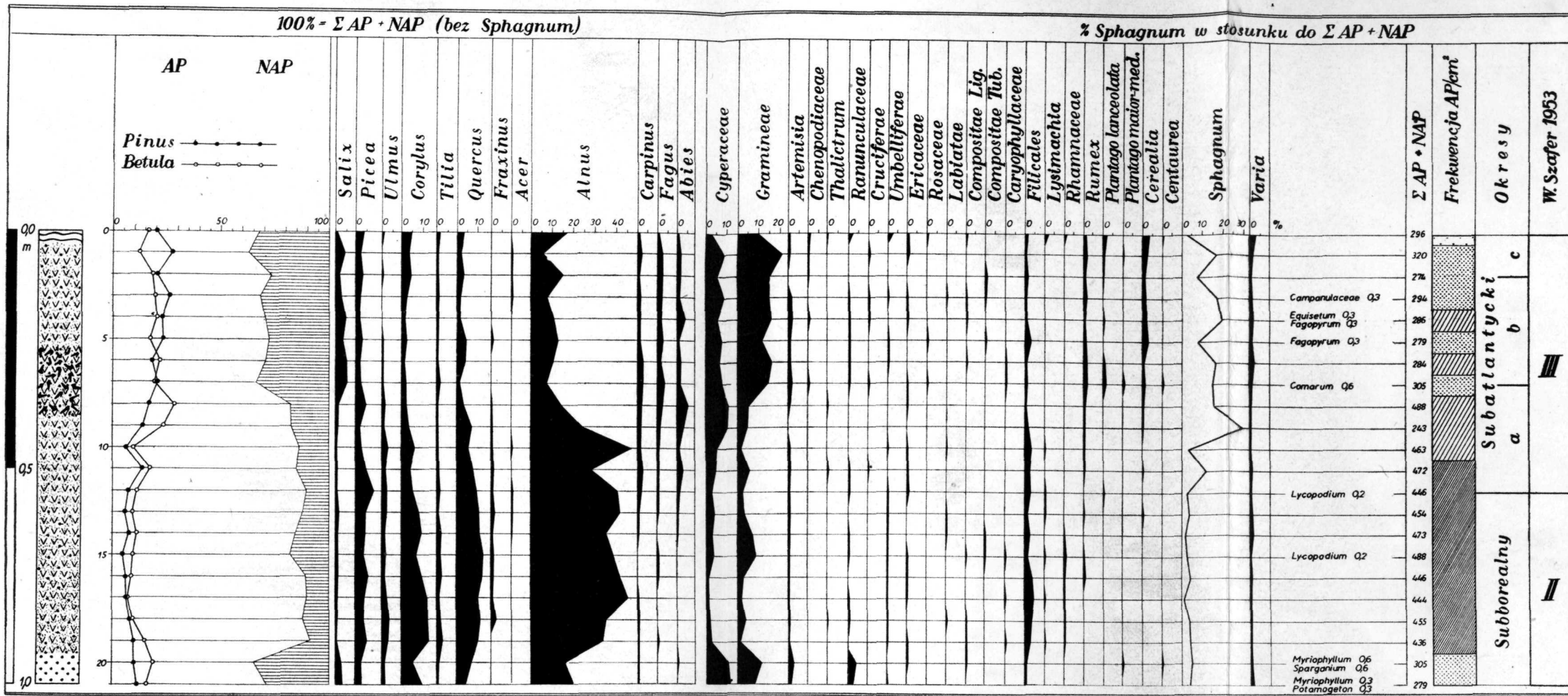
Ryc. 12. Diagram pyłkowy torfowiska Bodzentyn (300 m npm.)
