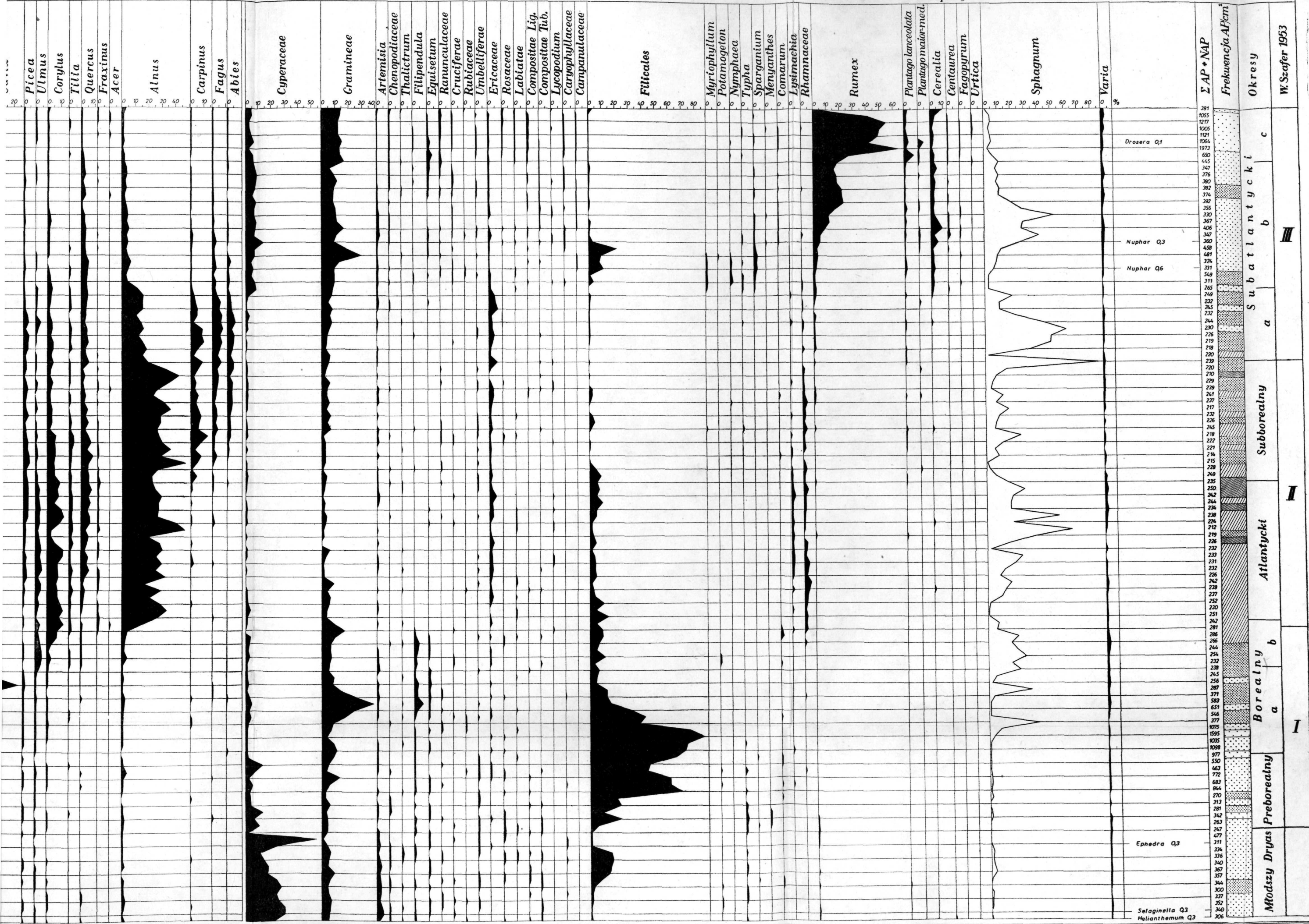
Ryc. 7. Diagram pyłkowy torfowiska Słopiec (250 m npm.) Fig. 7. Pollen diagram of the Słopiec peat bog (250 m a. s. l.)
