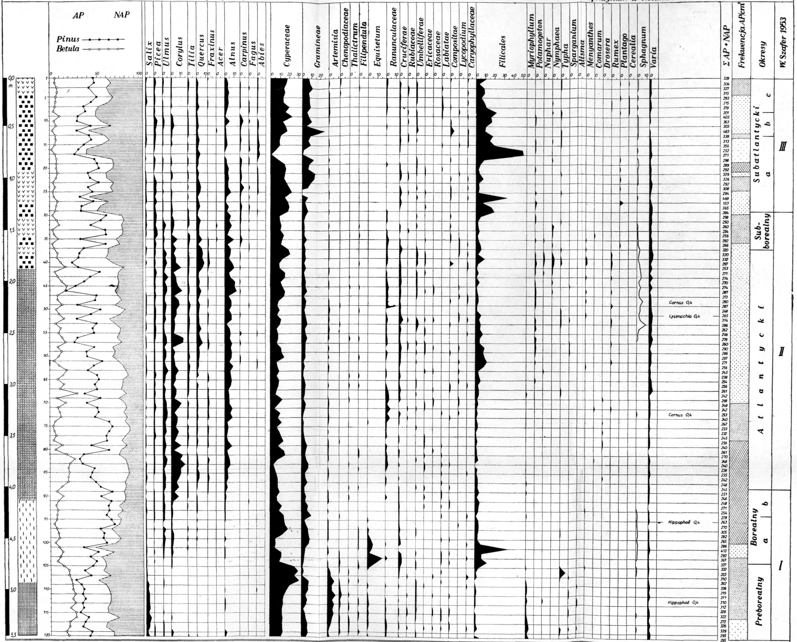
Ryc. 9. Diagram pyłkowy torfowiska Pakosław (188 m n.p.m.)
