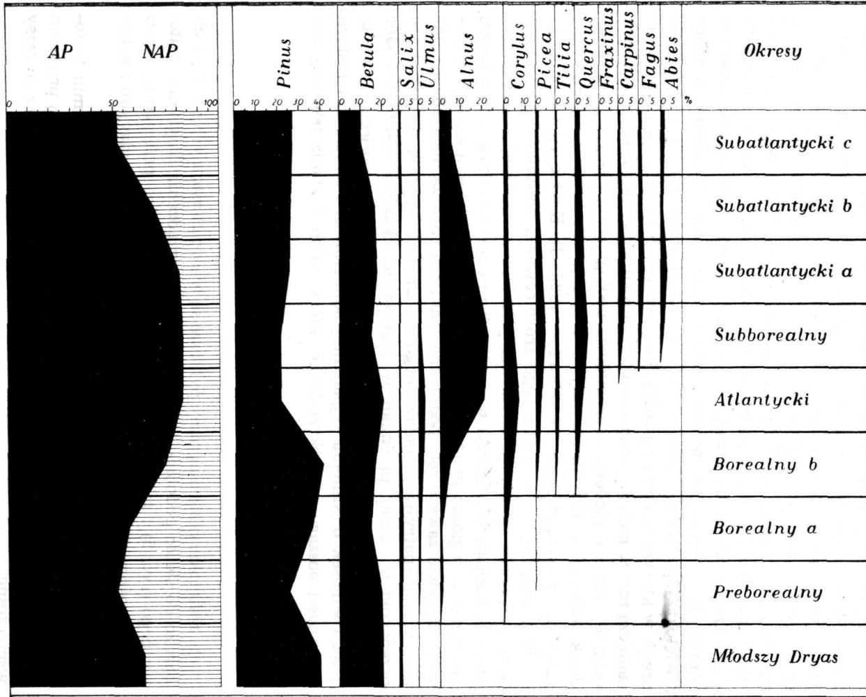
Ryc. 5. Syntetyczny diagram pyłkowy obrazujący przemiany w składzie lasów w późnym glacialu i holocenie Gór Świętokrzyskich
