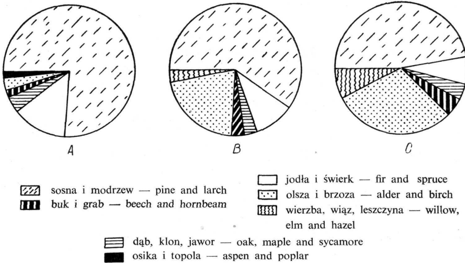
Ryc. 4. Cyclogramy przedstawiające A — procentowy skład współczesnych lasów województwa kieleckiego, B — procentowy udział pyłku drzew w próbach powierzchniowych, wyrażony jako średnie z siedmiu stanowisk, C — procentowy udział pyłku drzew występujących w podokresie „C” okresu subatlantyckiego, wyrażony jako średnie z siedmiu stanowisk
