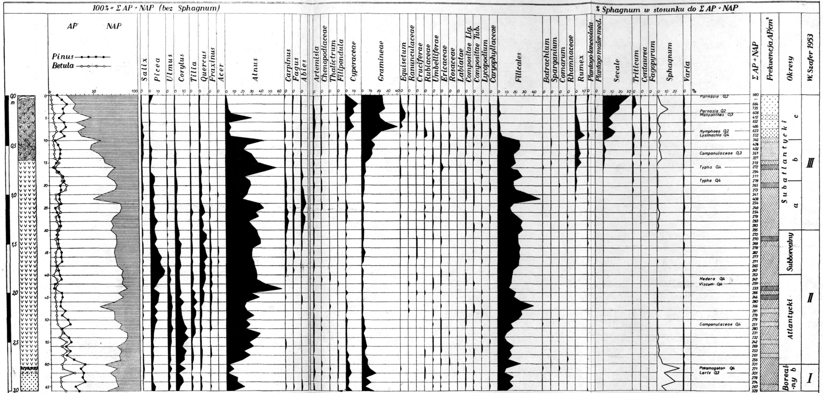
Ryc. 11. Diagram pyłkowy torfowiska Górno (240 m n.p.m.)
