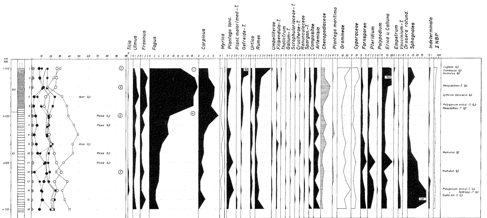
Abb. 22: Profil Nordstrandischmoor-III (NM-III). Über dem Torf liegen 58 cm Klei (Anwachs)
