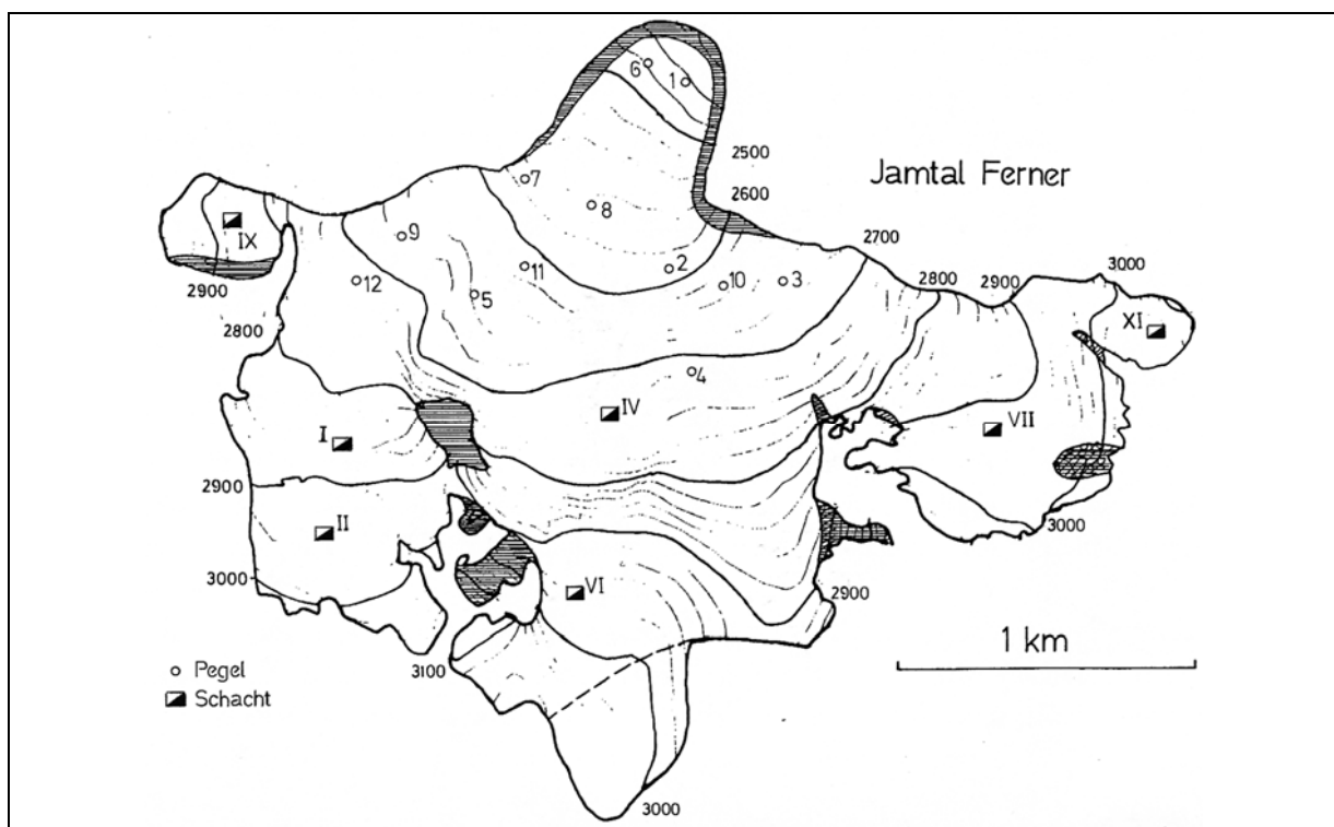
Abbildung 3: Lage der Schneeschnächte (Quadrate) und Pegel (Punkte) am Jamtal Ferner im April 2002. Die Messergebnisse sind in Tabelle 3 zusammengefasst.
