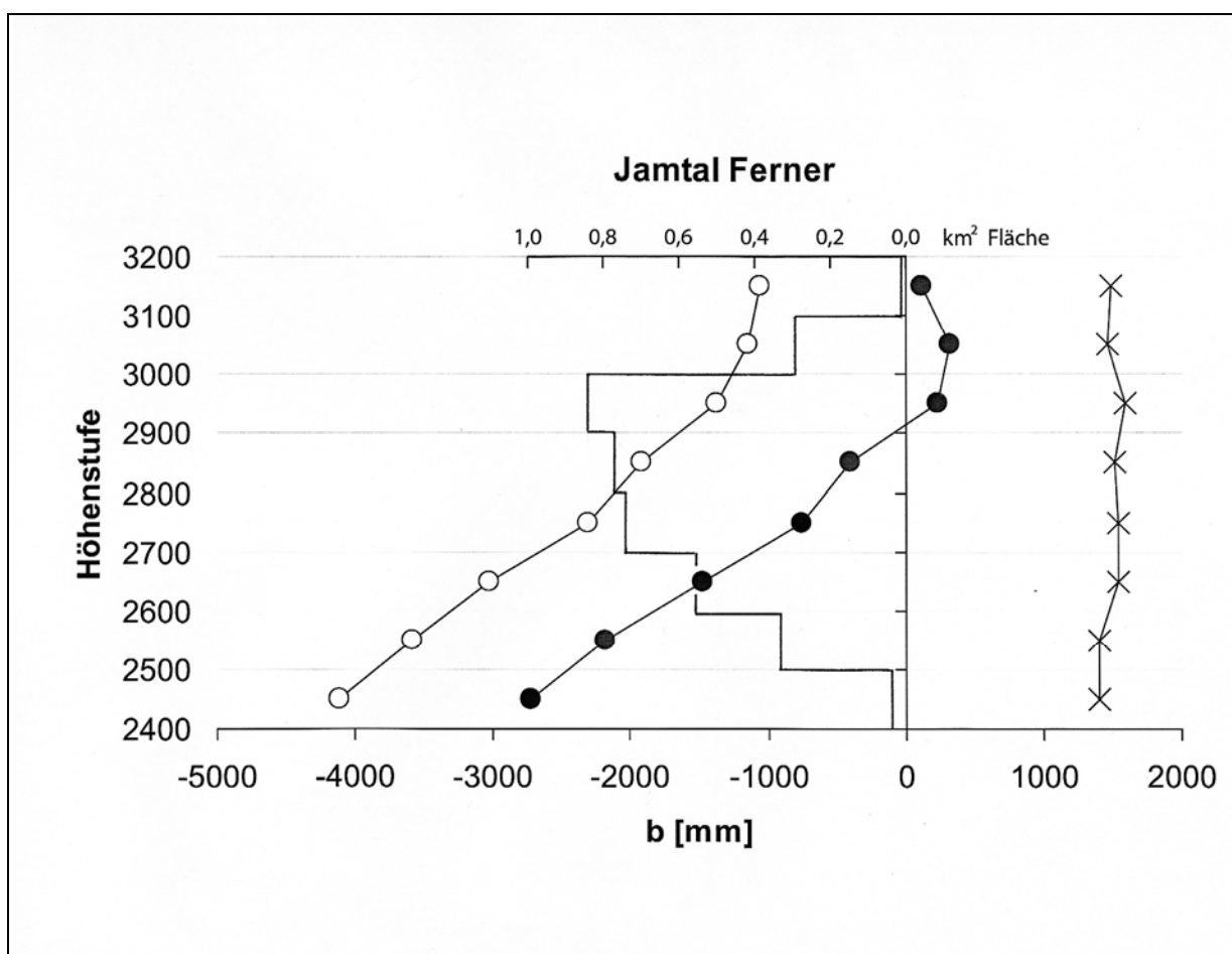
Abbildung 5: Die Verteilung der Flächen des Jamtal Ferners (durchgezogene Linie) und der Flächenmittel der spezifischen Jahresbilanz b (1.10.01 - 30.9.02 Punkte), der Winterbilanz b_{wj} (1.10.01 - 30.4.02 Kreuze) und der Sommerbilanz b_{so} (1.5. - 30.9.02 Kreise) für 100-m-Höhenstufen.
