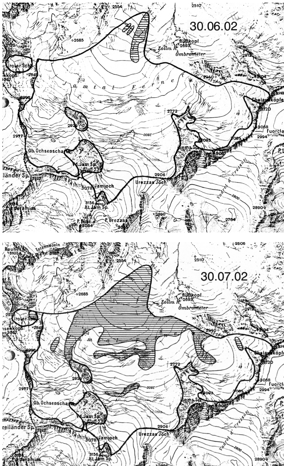
Abbildung 2: Die Schneebedeckung am Jamtal Ferner am 30.6. und 30.7.2002. Die schwarz schraffierten Flächen sind mit Altschnee bedeckt.
