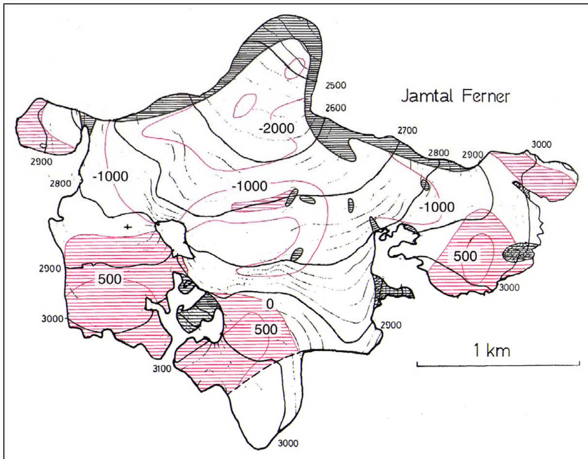
Abbildung 4: Isolinien des spezifischen Massenhaushaltes am Jamtal Ferner in mm Wasseräquivalent, gültig für den 30. 9. 2002. Die Flächen mit Nettoakkumulation sind rot schraffiert, die Teile des Gletschers, die seit der Kartenaufnahme abgeschmolzen sind, sind eng schraffiert.
