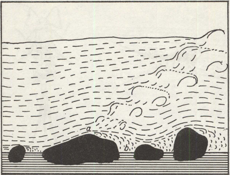
Bild 24: So entstehen Stillwasserzonen in der Strömung hinter Steinen. a leeseitige Abrißkante; b Still- oder Totwasserraum (nach AMBÜHL).
