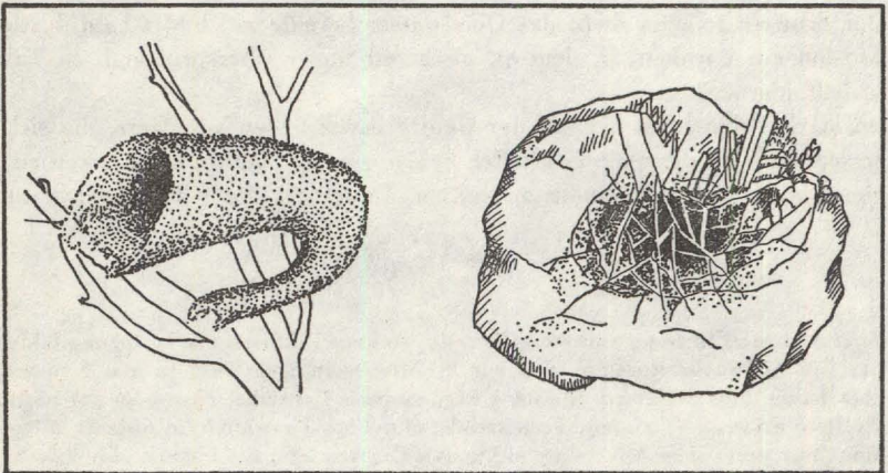
Bild 37: Reusen und Netze: Fangvorrichtungen verschiedener Köcherfliegenlarven.
