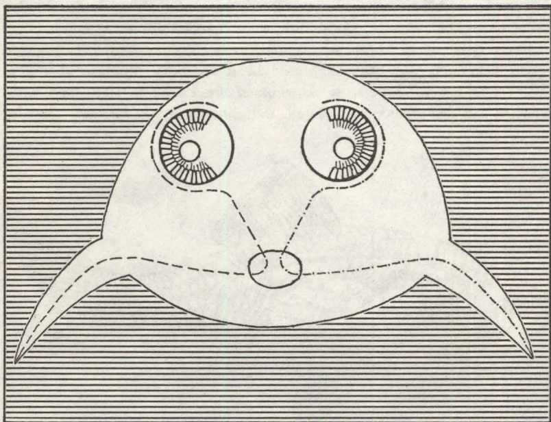
Bild 5: Prinzip eines Schwere-Sinnesorgans: Die schweren Steinchen drücken je nach Lage des Tieres auf immer wieder andere Sinneszellen, die diesen Reiz dem Zentralnervensystem melden.
