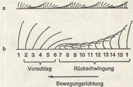
a Schlagfolge einer Wimperreihe; b Schlagphase einer Wimper. Aus MATTHES/WENZEL, Wimpertiere.
