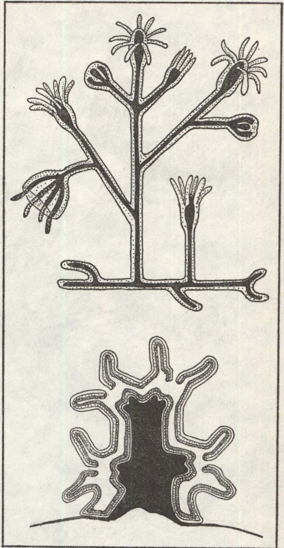
Bild 43: Bau eines Polypen- stockes und eines Korallen- stöckchens mit verkalkter Achse. Nach A. KÜHN.
