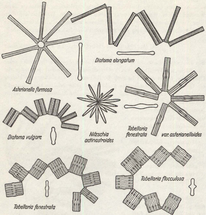
Bild 10: Sternförmige Kieselalgen aus dem Plankton. Kieselalgen sind einzellige Pflanzen mit einer Schale aus glasartiger, spröder Kieselsäure. Wir finden sie in allen Gewässern, vom Bergbach bis zum Ozean. So winzig auch die einzelne Zelle ist — durch ihre ungeheure Zahl können sie den Stoffhaushalt eines Gewässers dennoch nachhaltig beeinflussen. Sie sind pflanzliche, zur Photosynthese befähigte Lebewesen, die im Licht Sauerstoff produzieren und Kohlendioxid aus dem Wasser aufnehmen. Dadurch kann es zu einer Sauerstoffübersättigung kommen, aber auch — durch den Entzug der Kohlensäure — zu einer Alkalisierung des Wassers bis in Bereiche, die für empfindliche Tiere schädlich sind. Schalen von
